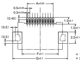
印刷基板加工尺寸 (顶视图)
