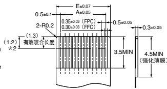
推荐FPC / FFC尺寸
